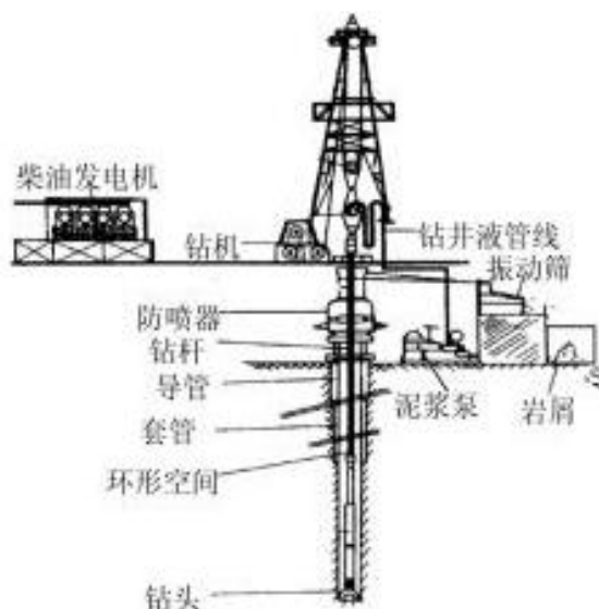
图2-7 钻井作业示意图
