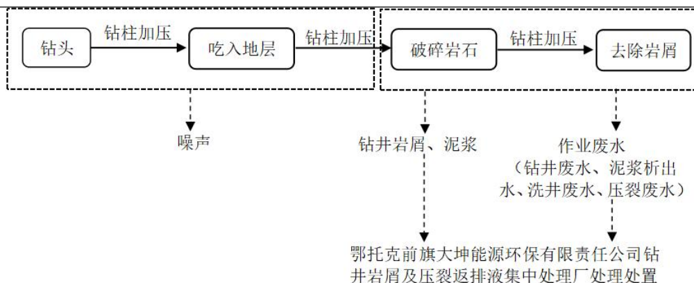
图 2-6 常规钻井工艺及产污环节图
