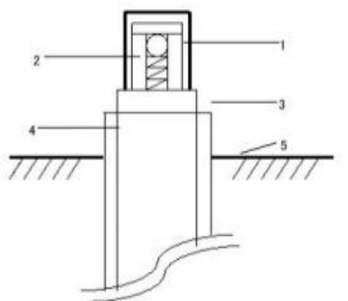
1-单流凡尔；2-钢板护罩；3-油管或接套；4-表套；5-地面
