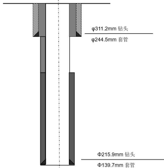
图 2-1 直井井身结构图
