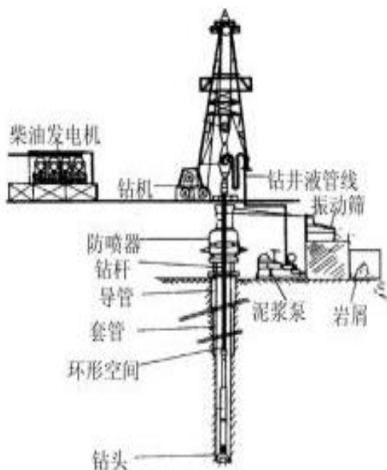
图2-7 钻井作业示意图
