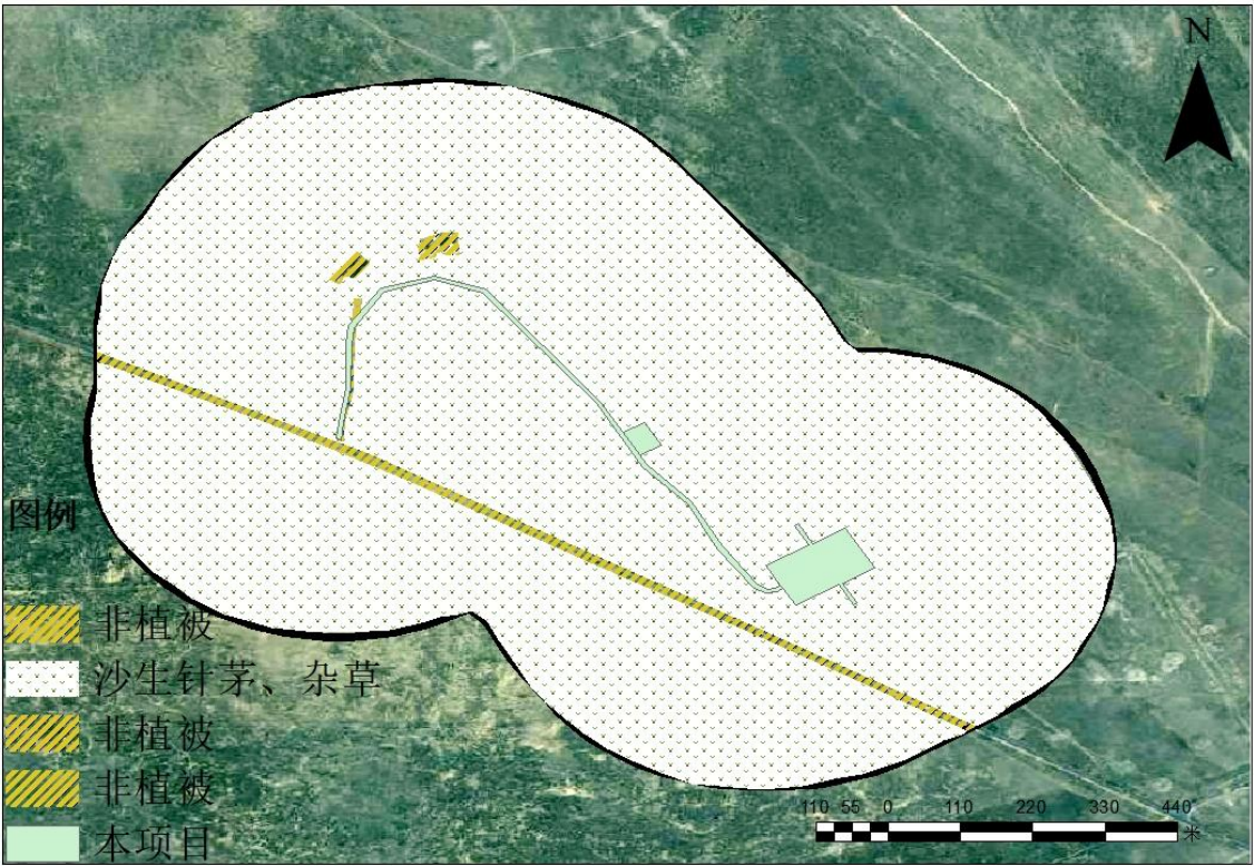
图 11 植被类型图
